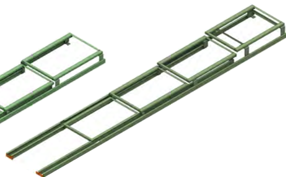
Conjunto para cinco tarimas en profundidad
