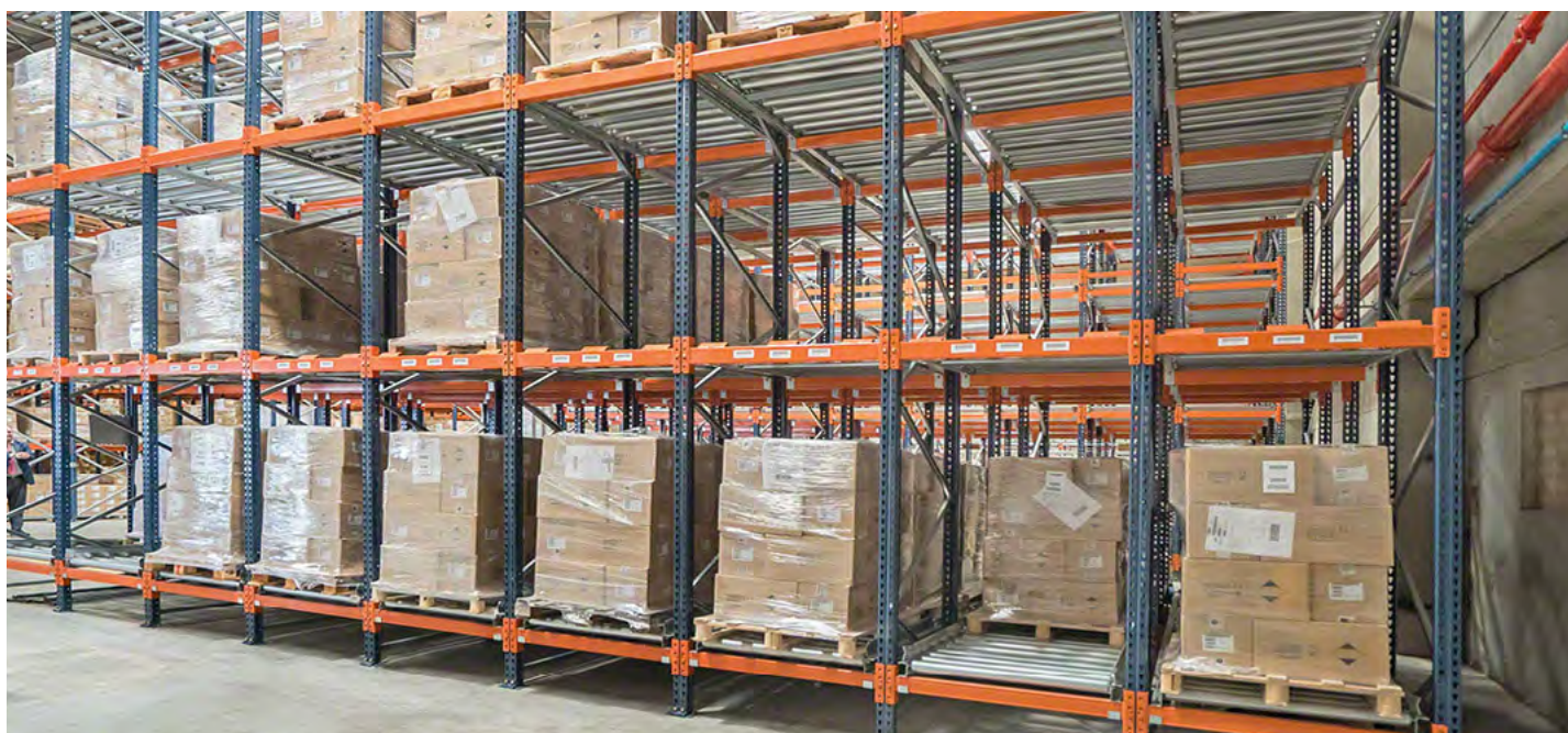
Tope/retén de tarimas
