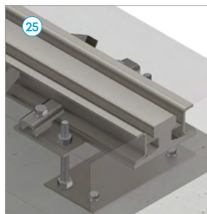
Carril guía
