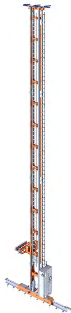
Transelevador monocolumna MLHP Alcanza los 21 m de altura y puede transportar dos unidades de carga de 50 kg cada una.
