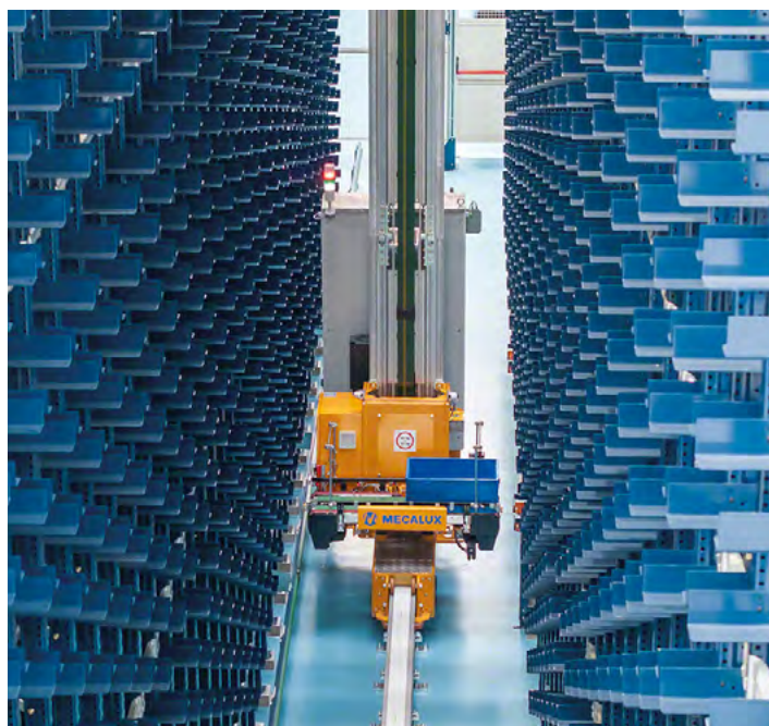
Transelevador bicolumna MLB100Q Capaz de alcanzar los 20 m de altura y transportar dos unidades de carga (de 100 kg cada una) o cuatro de 50 kg.
